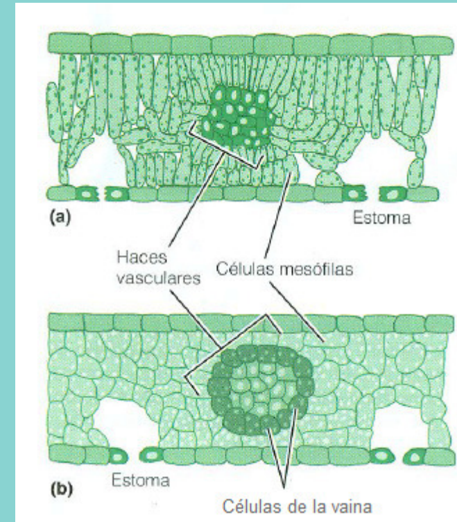
Fig.1: Anatomía foliar de plantas C 3 y C 4
